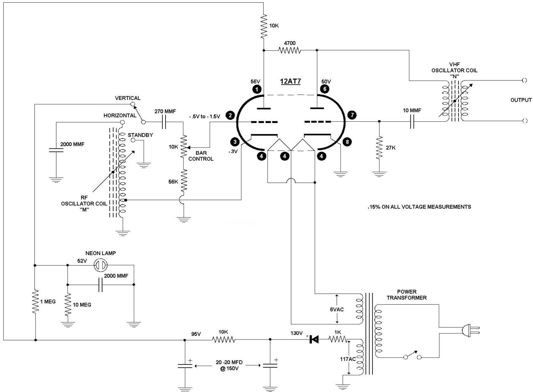
HEATHKIT BAR GENERATOR
