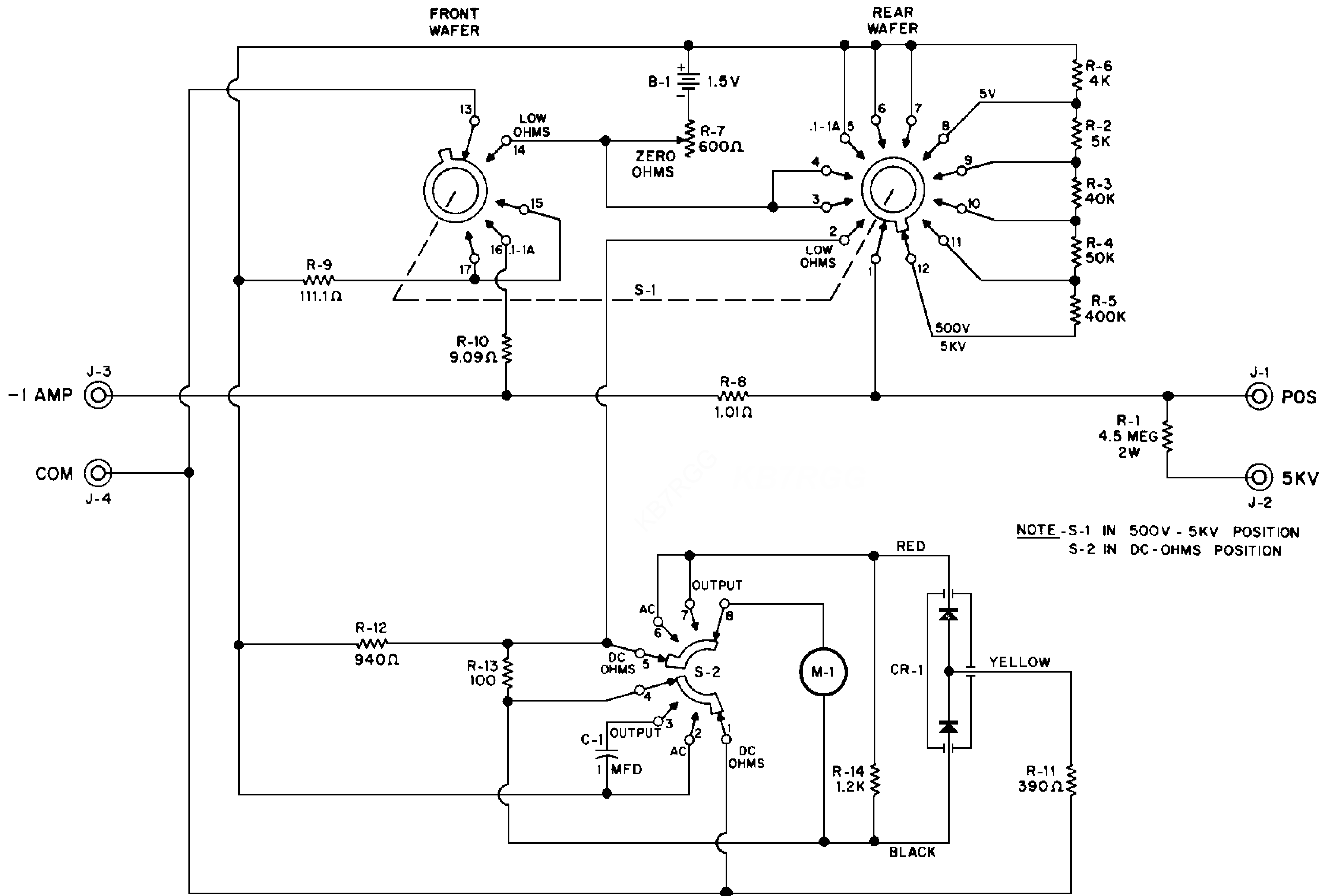
knight-kit 1000 Ohms/Volt VOM
